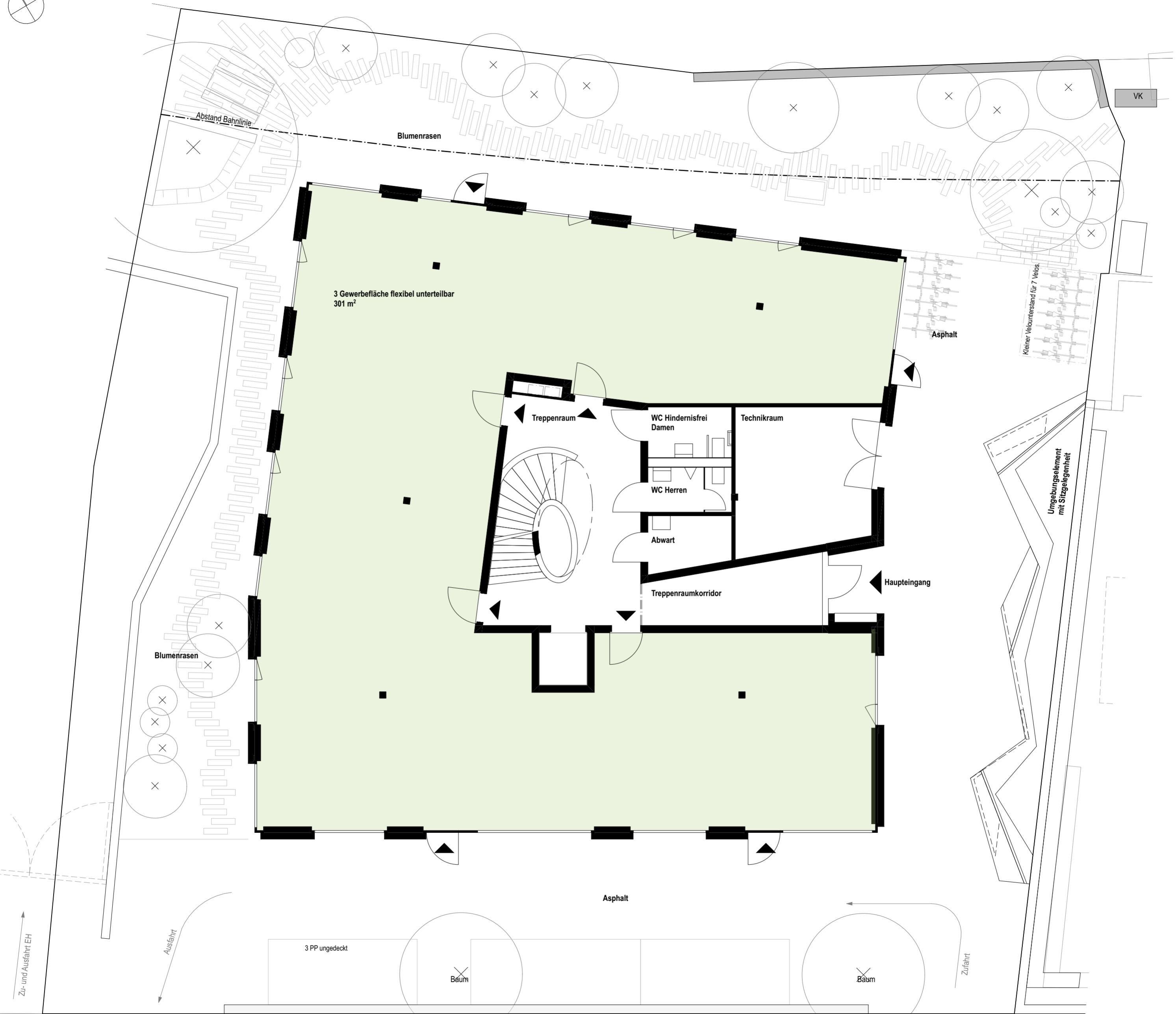
Grundriss Erdgeschoss 1:100
